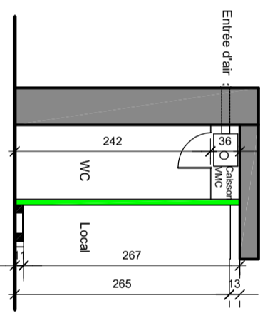
COUPE B-B
