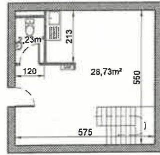
Sous-Sol
